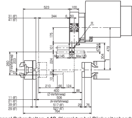
3295-H280 (Doppel-Bohrerhalter: \phi 40 (Korrektur bei Rückseitenbearbeitung)) *Keine Werkzeuge für Rückseitenbearbeitung an der inneren Werkzeugposition.
