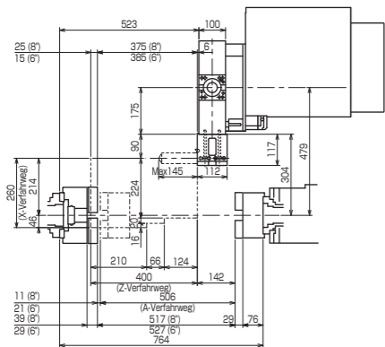
3295-H230 (Bohrerhalter für Vorderseitenbearbeitung: \phi 40 )
