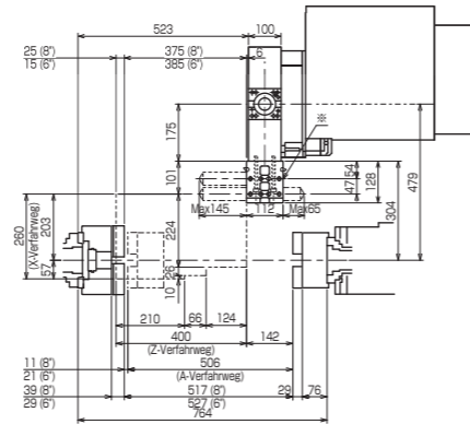
3295-H220 (Doppel-Bohrerhalter: \phi 40 ) *Keine Werkzeuge für Rückseitenbearbeitung an der inneren Werkzeugposition.
