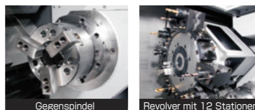
Gegenspindel Revolver mit 12 Stationen
