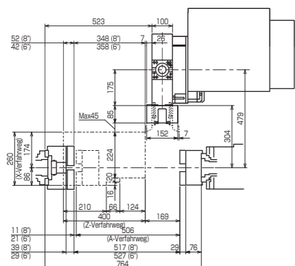
3295-H210 (Doppel-Drehwerkzeughalter)
