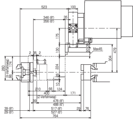
3295-H250 (Abstechwerkzeughalter)
