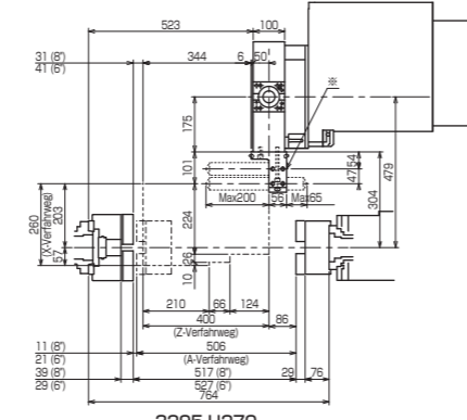
3295-H270 (Doppel-Bohrerhalter: \phi 40 (Korrektur bei Vorderseitenbearbeitung)) *Keine Werkzeuge für Rückseitenbearbeitung an der inneren Werkzeugposition.
