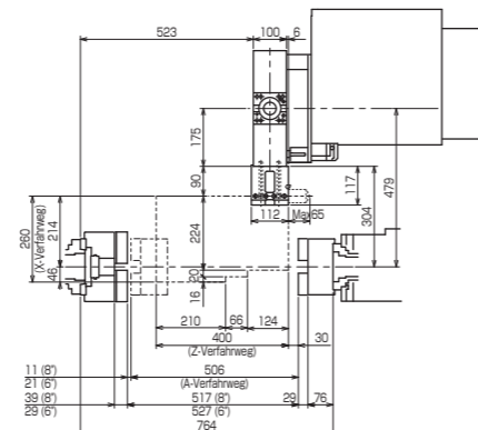
3295-H240 (Bohrerhalter für Rückseitenbearbeitung: \phi 40 )
