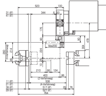
3295-H290 (Bohrerhalter für Vorderseitenbearbeitung: \phi 40 (Korrektur bei Vorderseitenbearbeitung))
