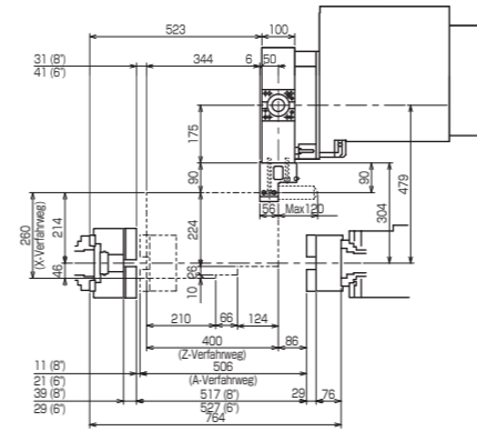
3295-H300 (Bohrerhalter für Rückseitenbearbeitung: \phi 40 ) (Korrektur bei Rückseitenbearbeitung)
